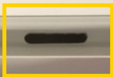
Reparatur / Abdichtung von Entwässerungsöffnungen
